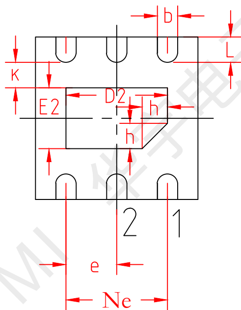
背视图
