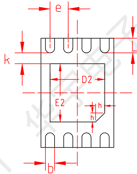
BOTTOM VIEW 背视图
